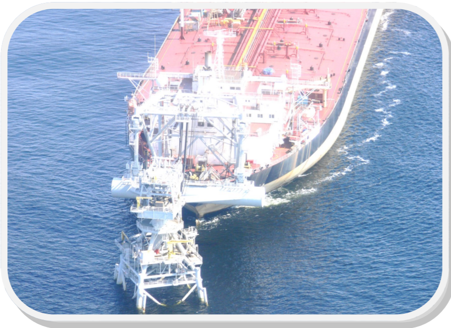
Une vue du Terminal Komé-Kribi 1 du Pipeline Tchad/Cameroun
